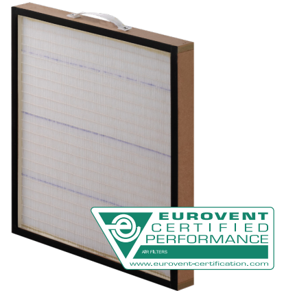
VariPak 592x592 mm
